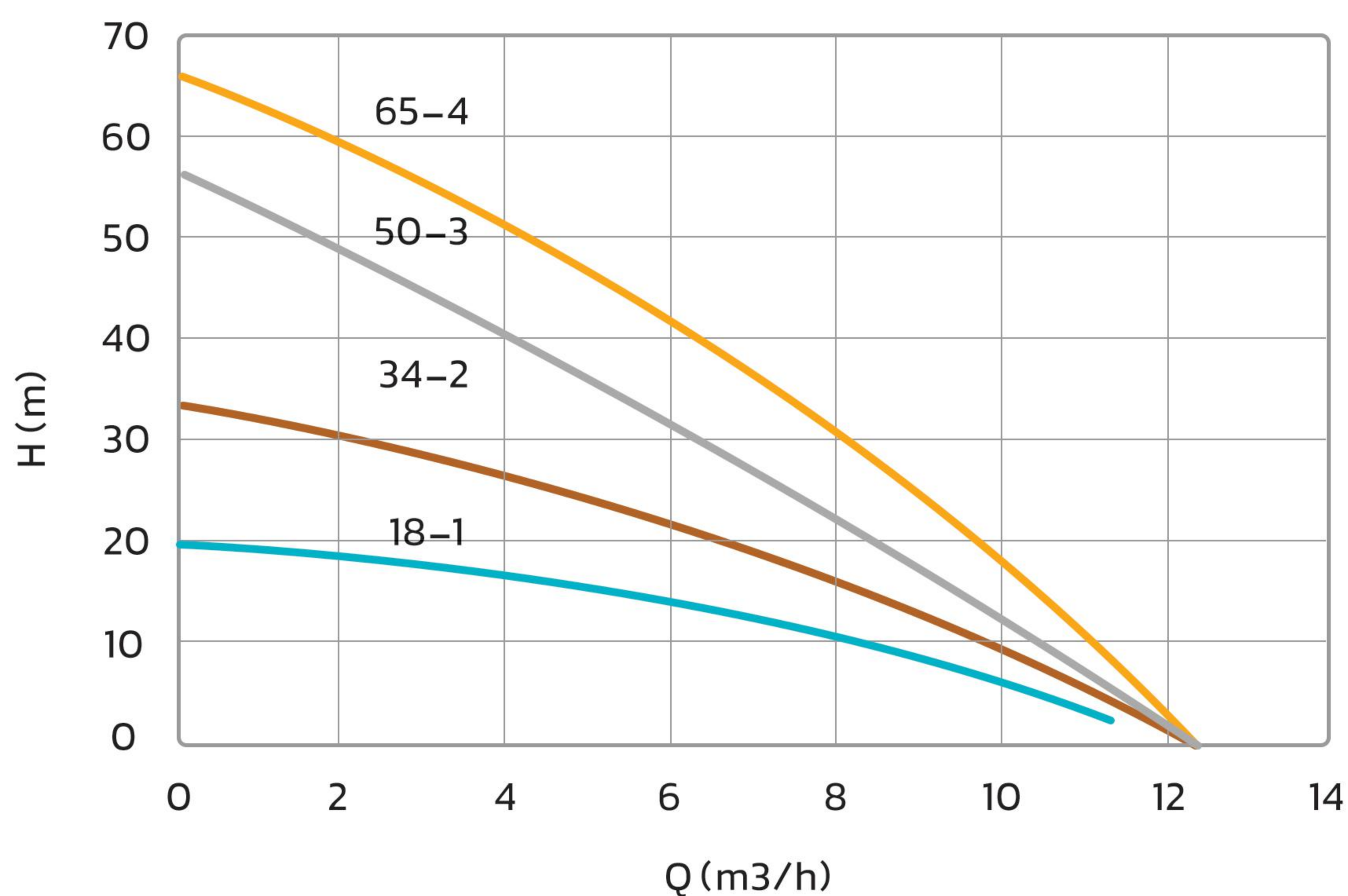
جدول مشخصات فنی و ابعادی الکتروپمپ‌ها Technical and dimensional specifications table for electropumps
