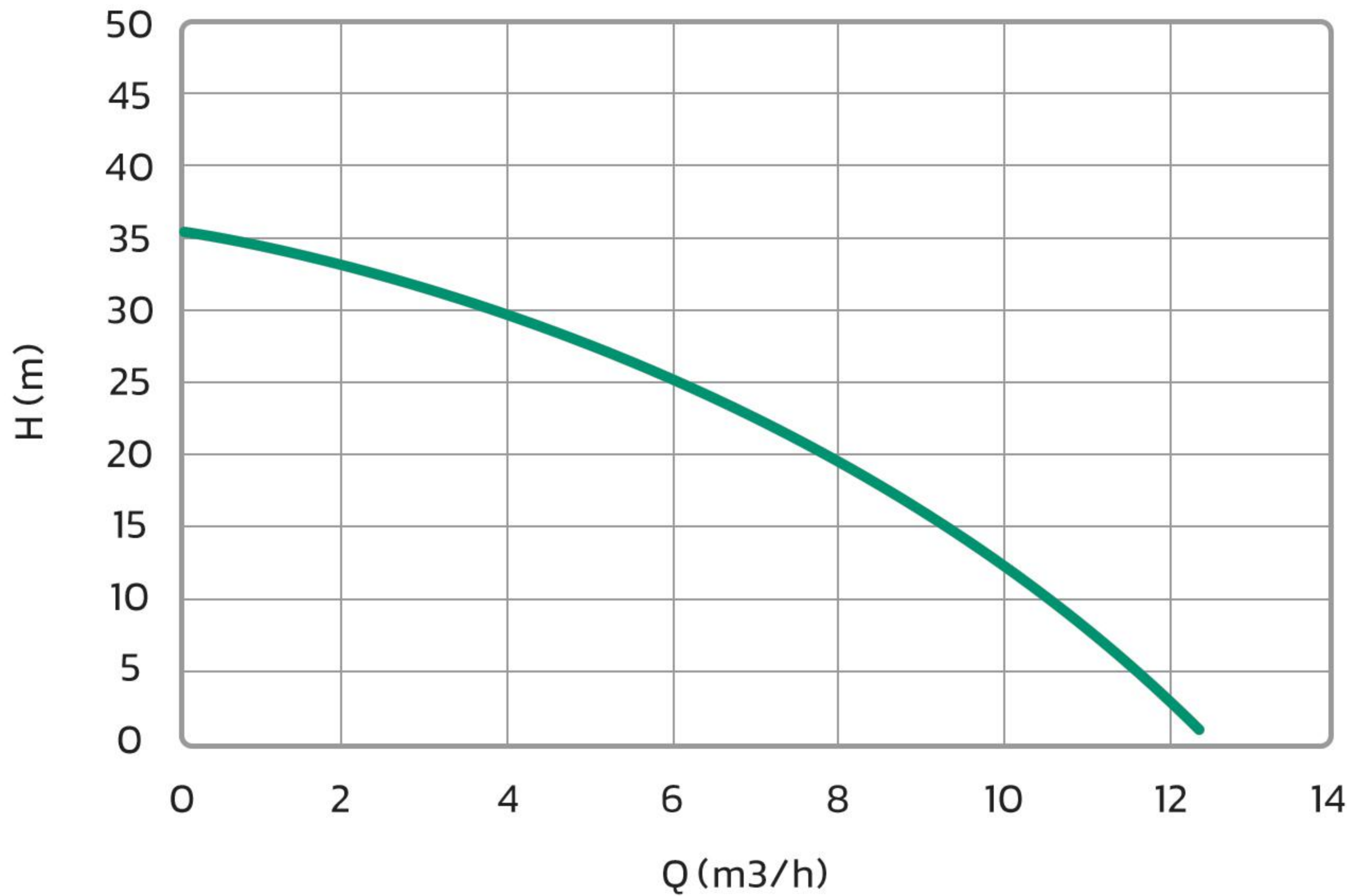
منحنى الكترورمپ Electropump Curve
